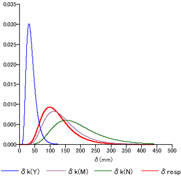
各損傷(C,Y,M,N)および応答(Resp)の確率密度関数(対数正規分布)
