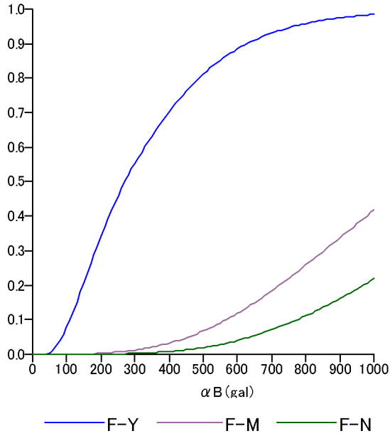
各損傷レベルの限界状態発生累積確率関数
