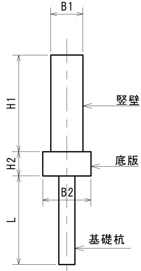
下部工側面図
