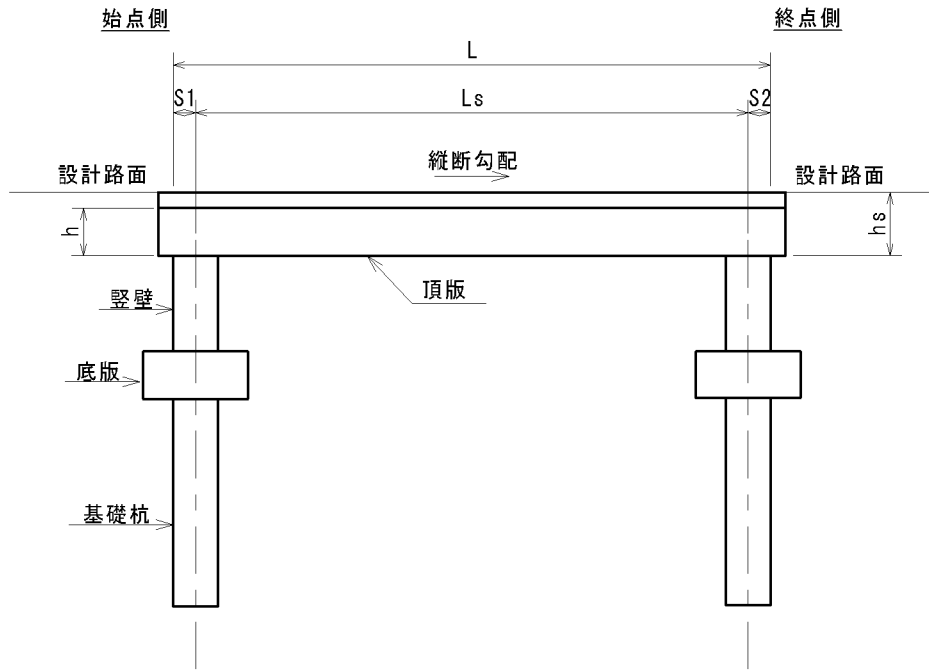
橋梁側面図
