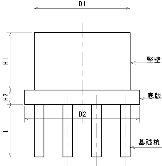
下部工正面図
